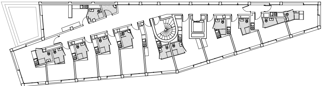
Plan de l'étage R+4
