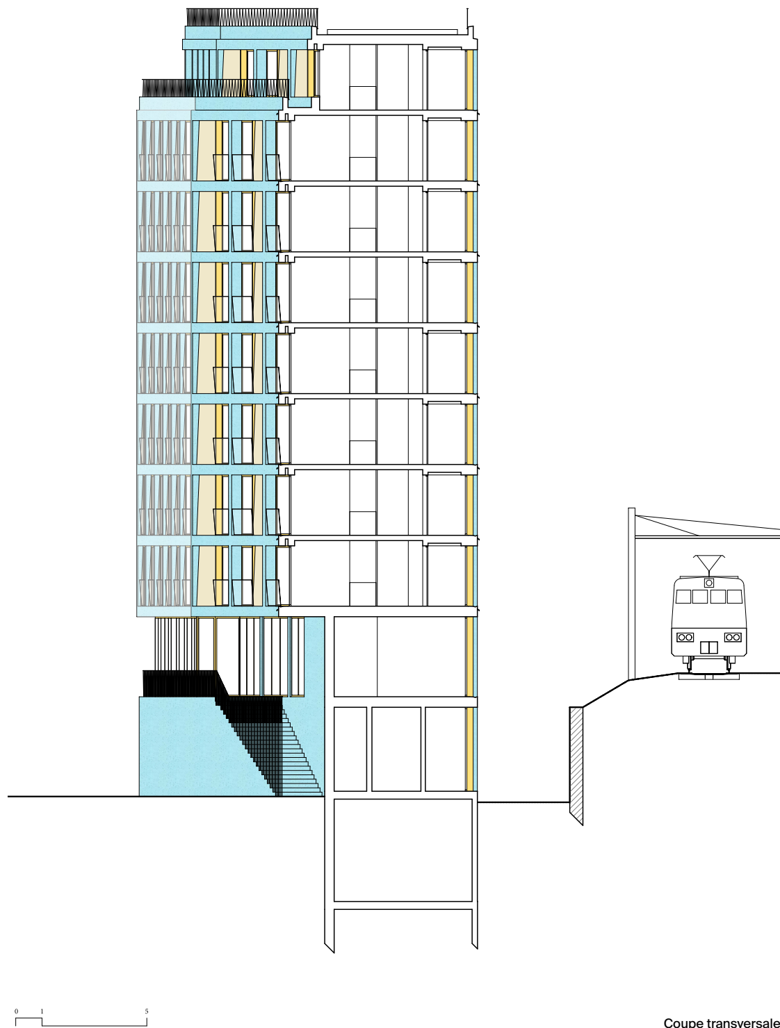
Coupe transversale
