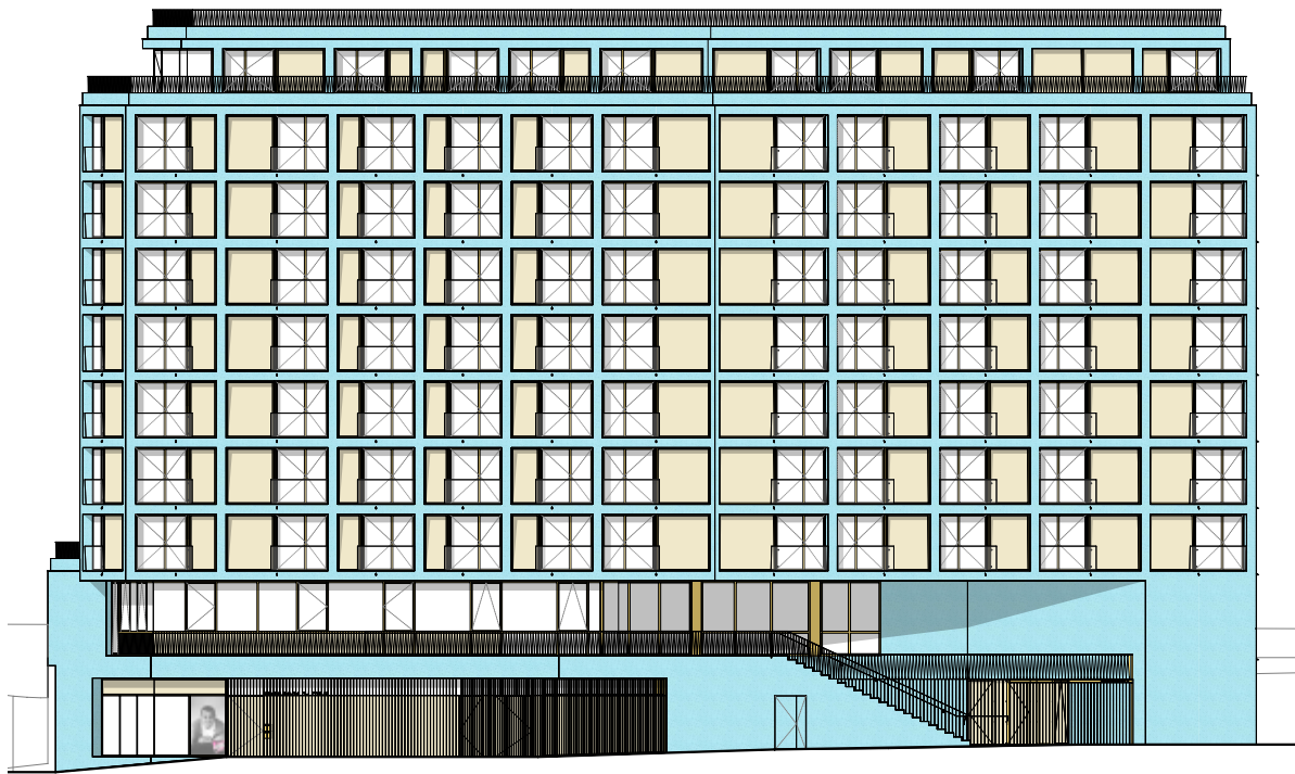
Élévation Est
