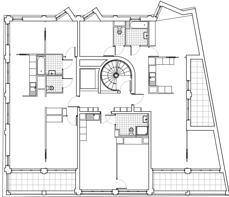
Plan de l'étage R+1
