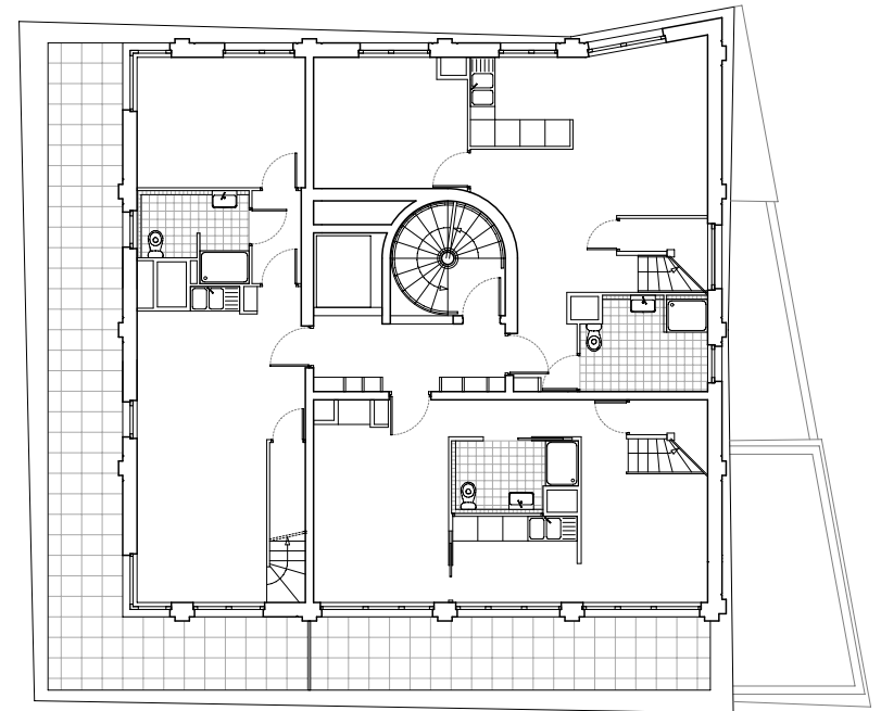
Plan de l'étage R+7
