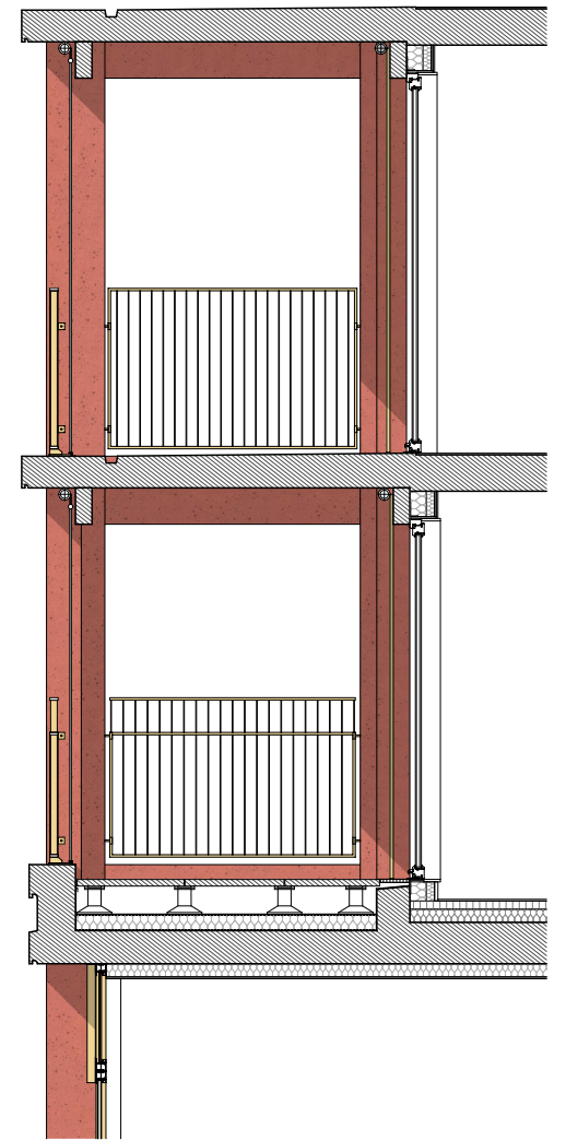
Détail de façade
