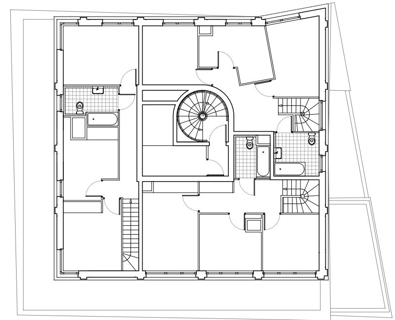
Plan de l'étage R+8
