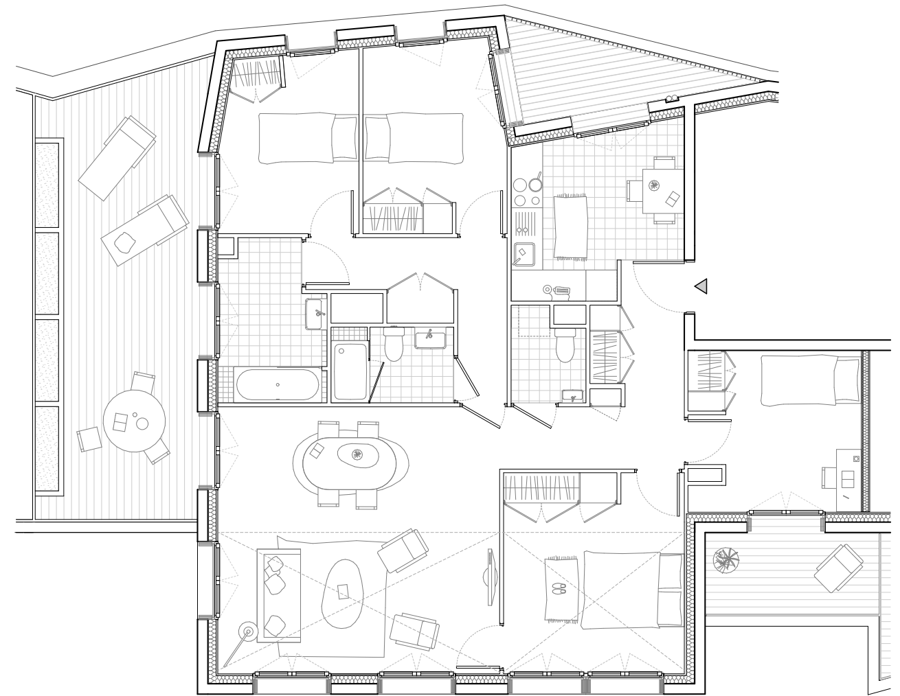
Plan d'un logement T5
