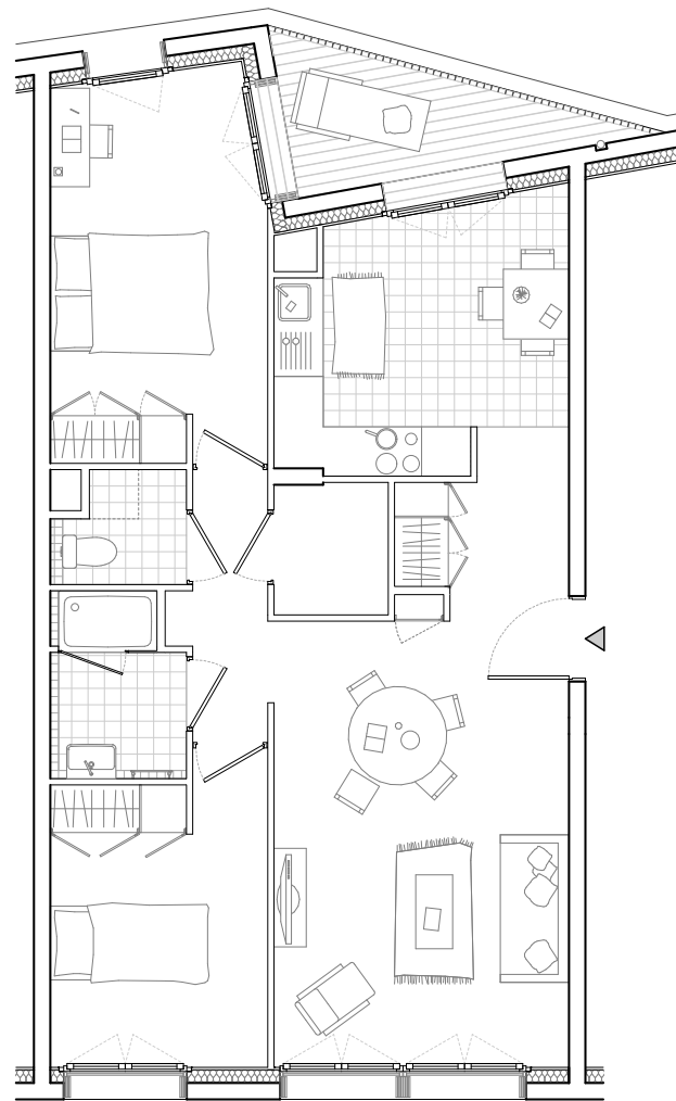
Plan d'un logement T3
