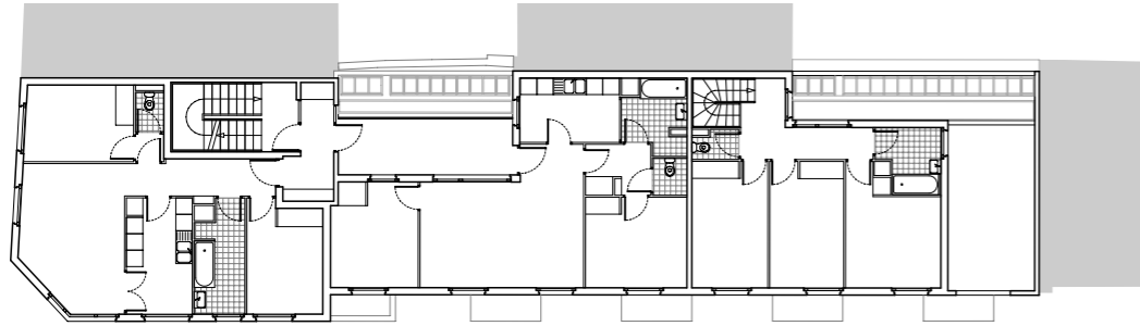
Plan de l'étage R+2
