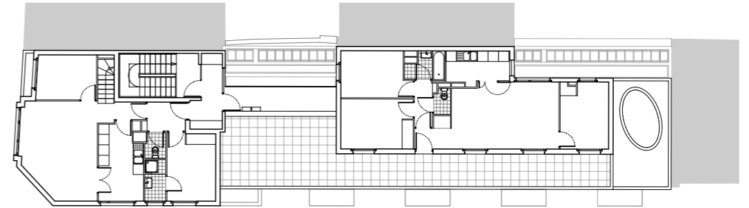
Plan de l'étage R+3
