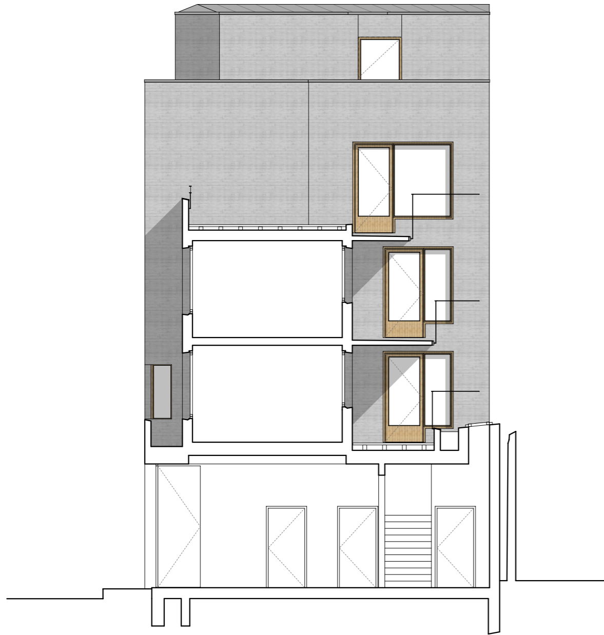
Coupe transversale
