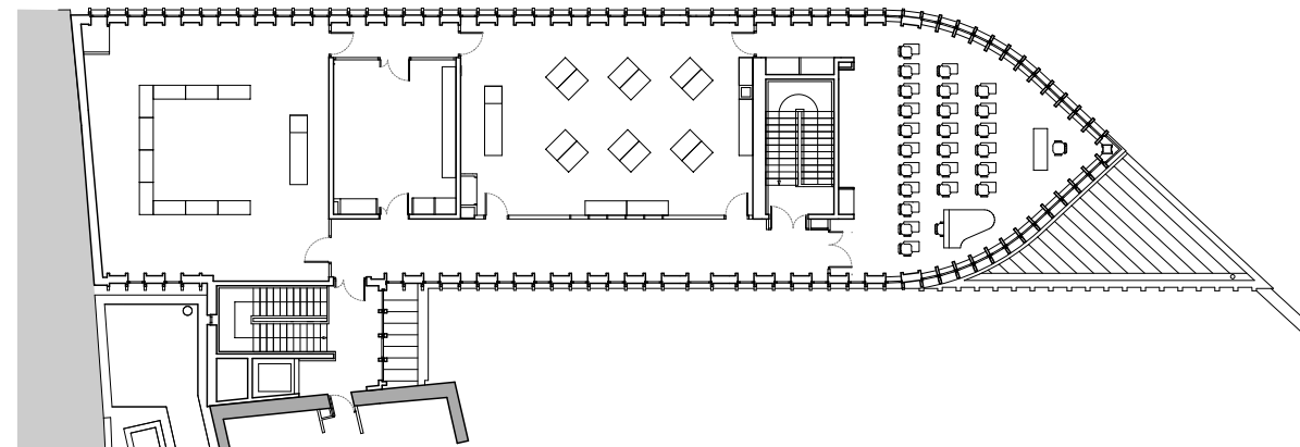
Plan de l'étage R+2
